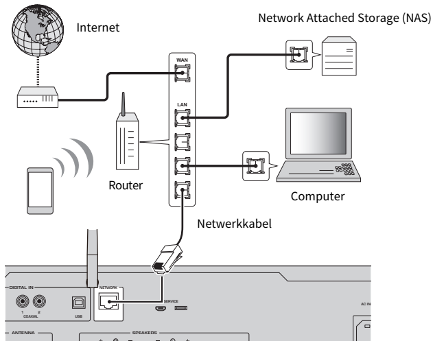
Achterpaneel
