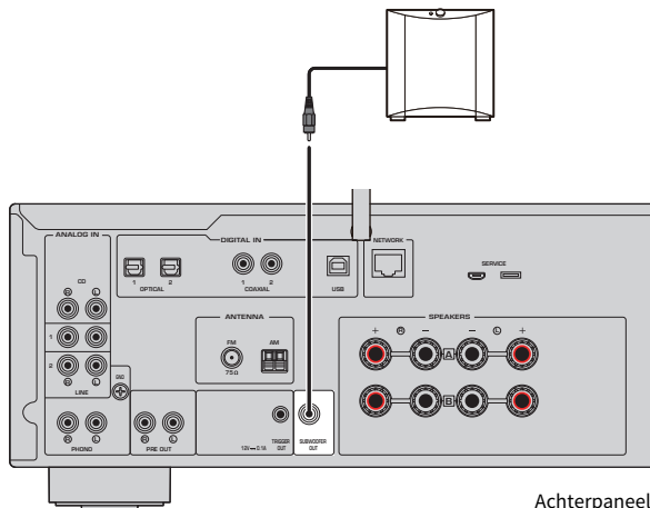
Achterpaneel
