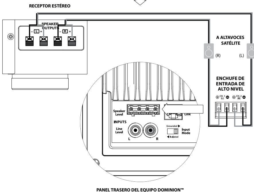
PANEL TRASERO DEL EQUIPO DOMINION™
