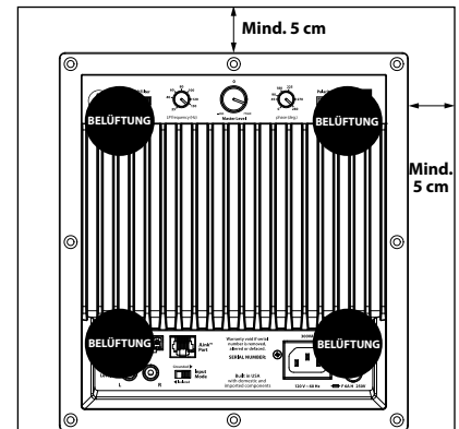
Rückansicht bei Gehäuseeinbau:
