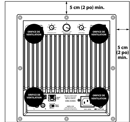
Vue arrière du boîtier :
