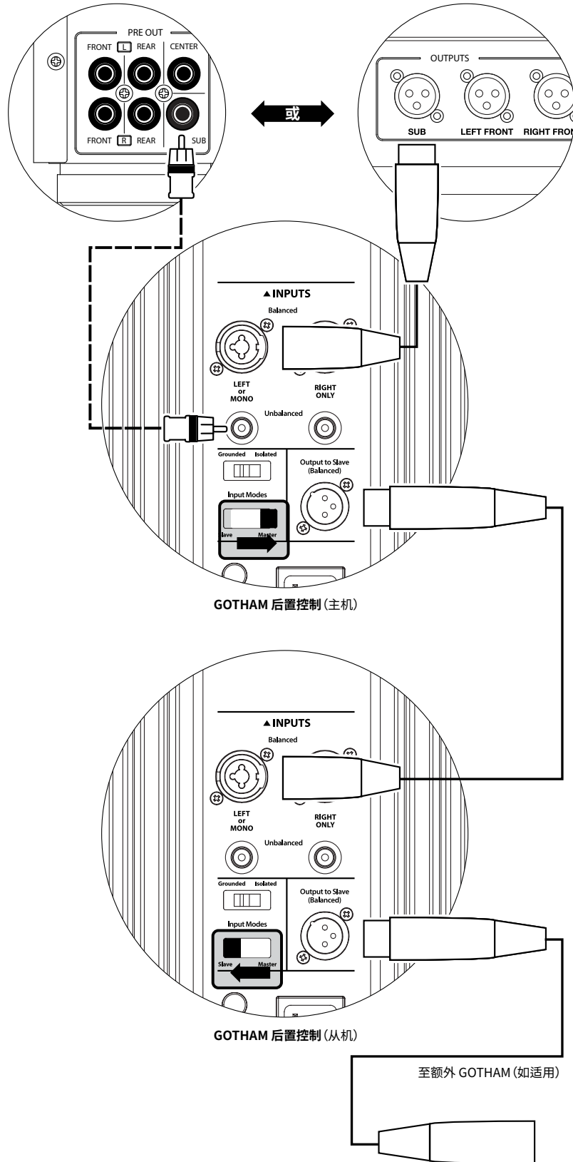
接收器/处理器 (非平衡输出)
