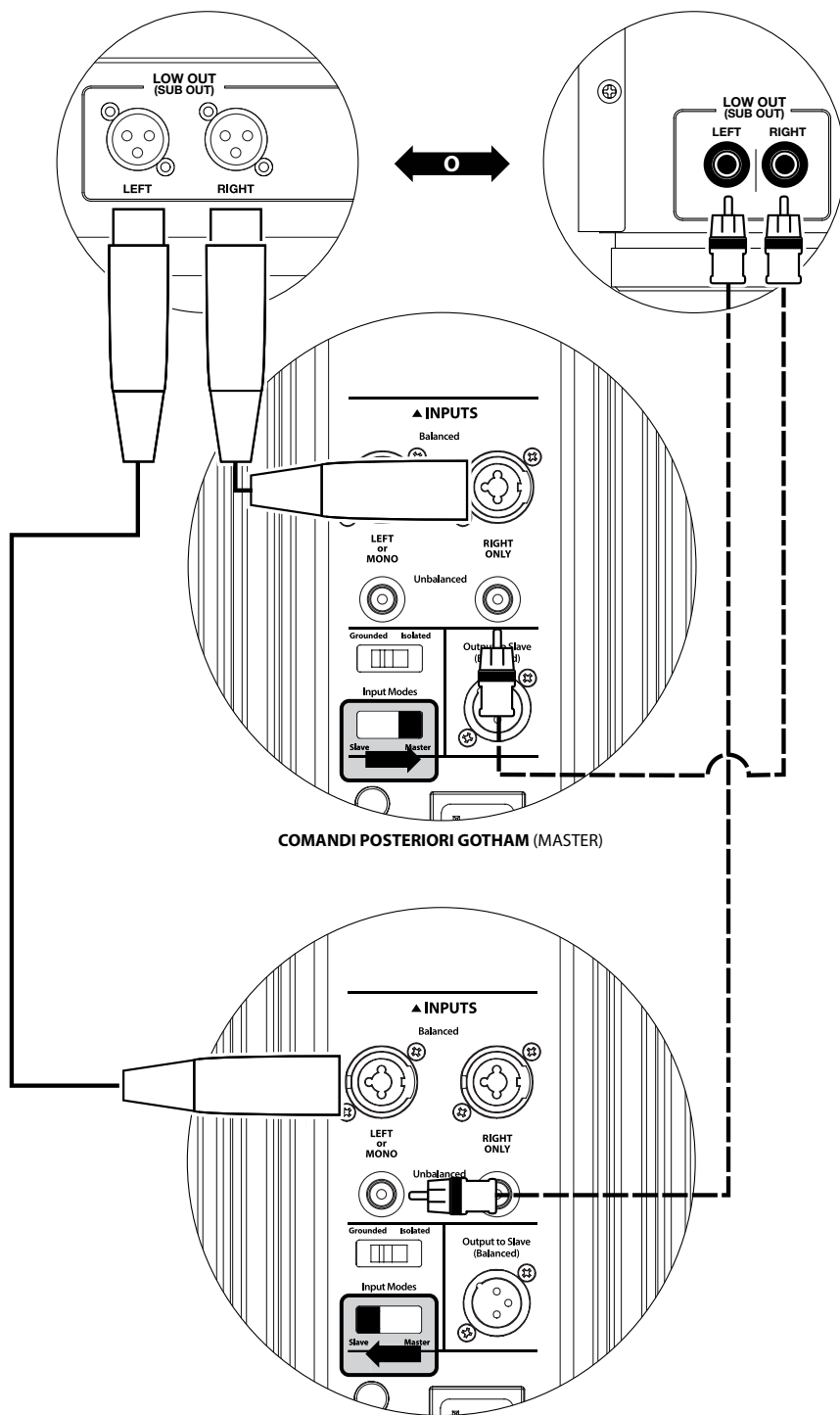
CROSSOVER ATTIVO STEREO (USCITE BILANCIATE)
