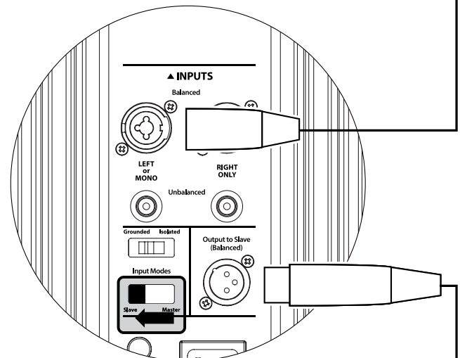
GOTHAM HINTERE BEDIENELEMENTE (SLAVE)
