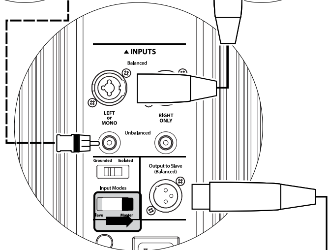
GOTHAM HINTERE BEDIENELEMENTE (MASTER)
