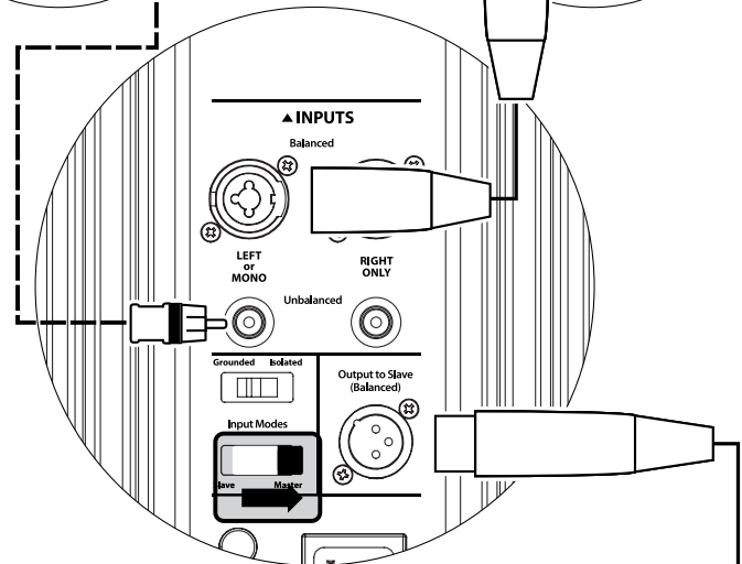
BOUTONS DE RÉGLAGE ARRIÈRE DU GOTHAM (MAÎTRE)
