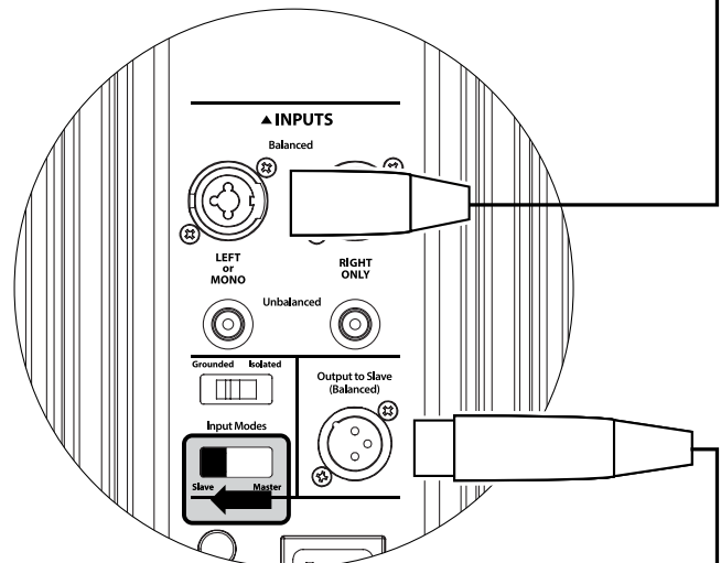
BOUTONS DE RÉGLAGE ARRIÈRE DU GOTHAM (ESCLAVE)
