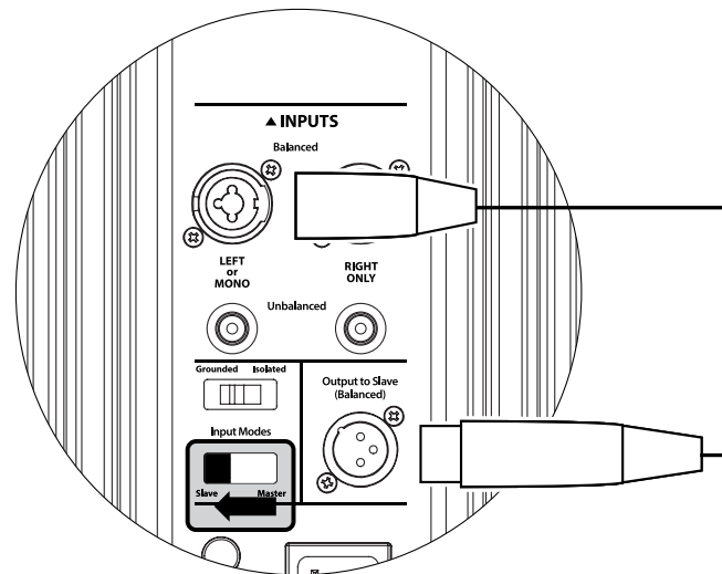
COMANDI POSTERIORI GOTHAM (SLAVE)
