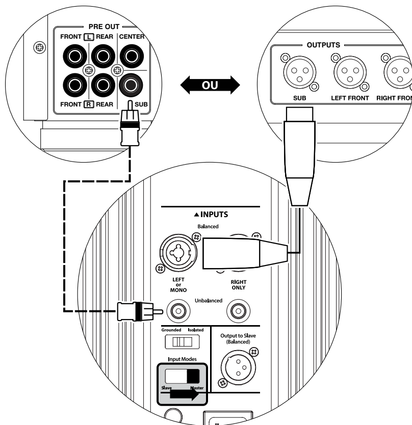
BOUTONS DE RÉGLAGE ARRIÈRE DU GOTHAM (MAÎTRE)
