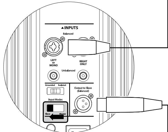
CONTROLES TRASEROS GOTHAM (ESCLAVO)
