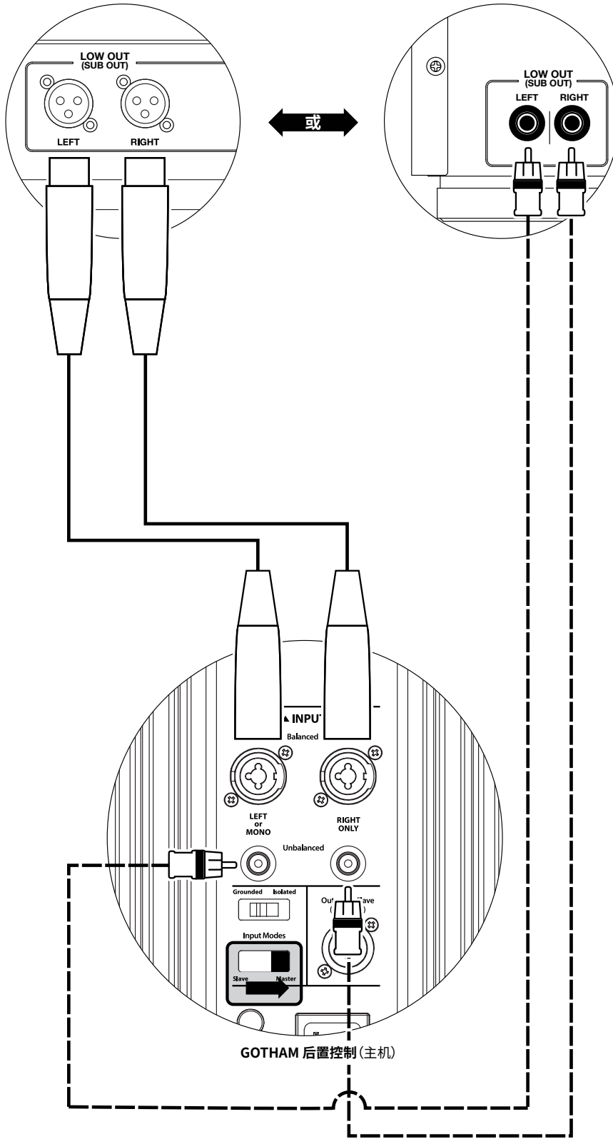
立体声有源分频器 (平衡输出)
