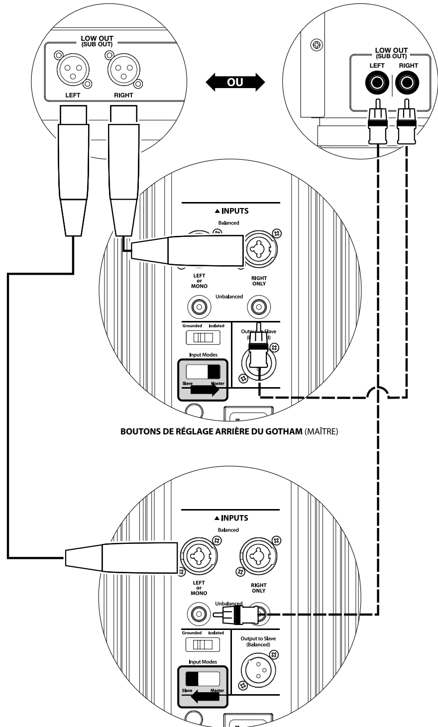
FILTRE ACTIF STÉRÉO (SORTIES SYMÉTRIQUES)
