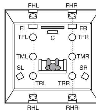
[Bovenaanzicht]
