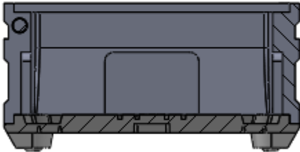
SCHNITT A-A
